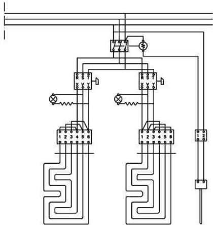
TOP Kw 2,4
